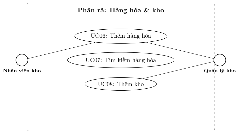
Figure 1: Use case phân rã – Hàng hóa và kho
